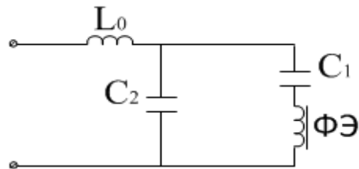
Fig.4. PITSIM scheme
