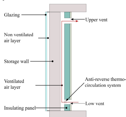
Fig. 1. A composite Trombe wall.
